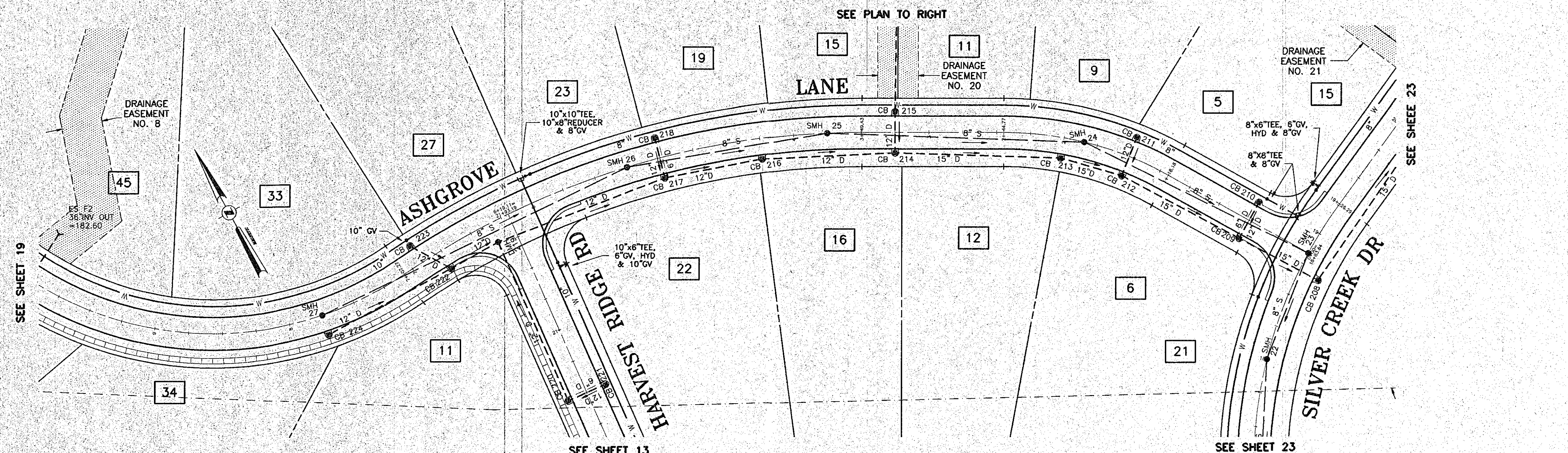
1 PLAN - ASHGROVE LN STA 0+00 TO STA 9+75 SCALE: 1" = 50' CROSS REFERENCE: NONE
