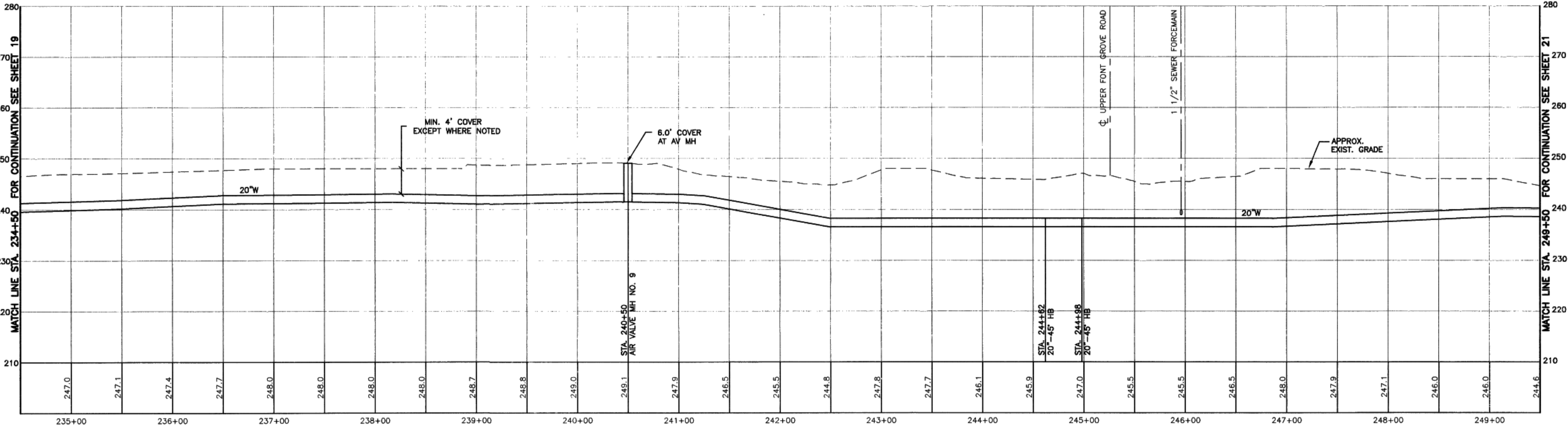
PROFILE SCALE: (HORIZ.) 1"=50' (VERT.) 1"=10'
