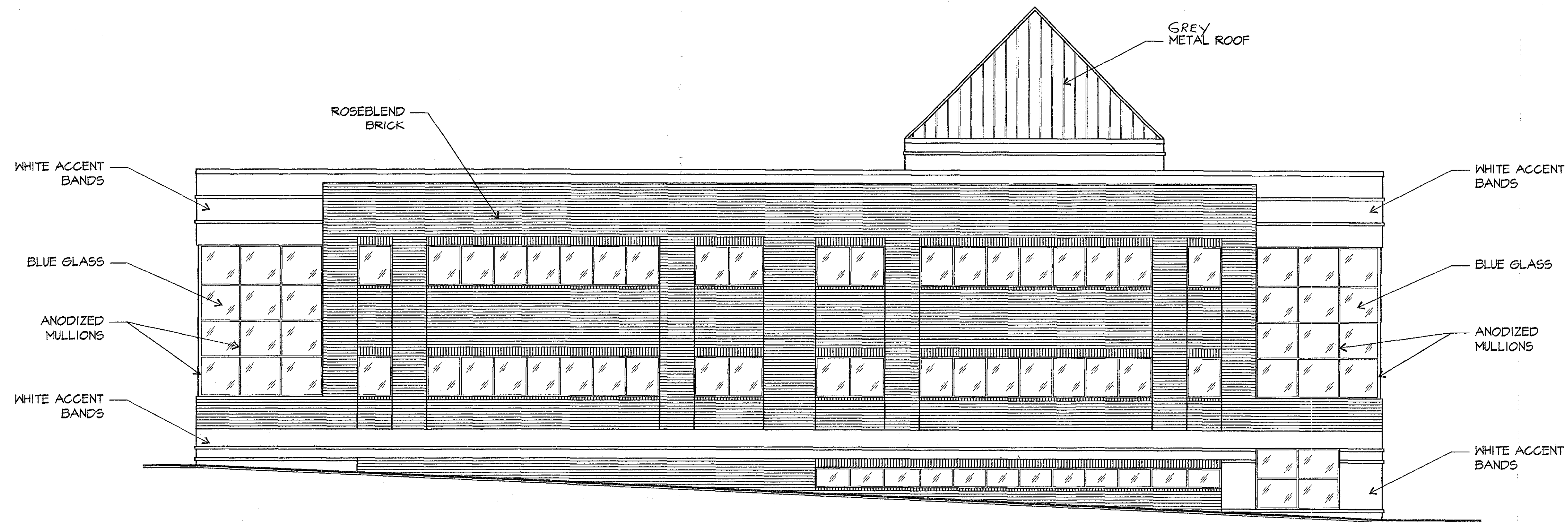
1 A-4 SIDE ELEVATION
