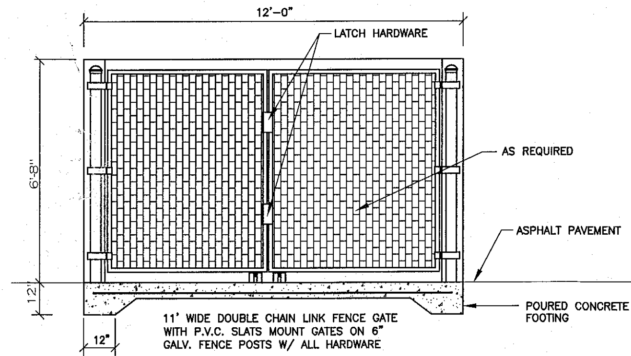
ELEVATION B
