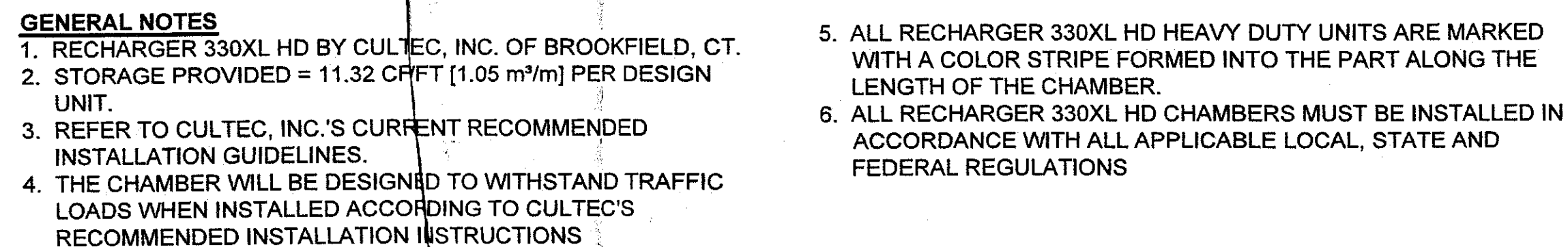
4 CULTEC R330 XLHD STORM CHAMBER SCALE: N.T.S.
