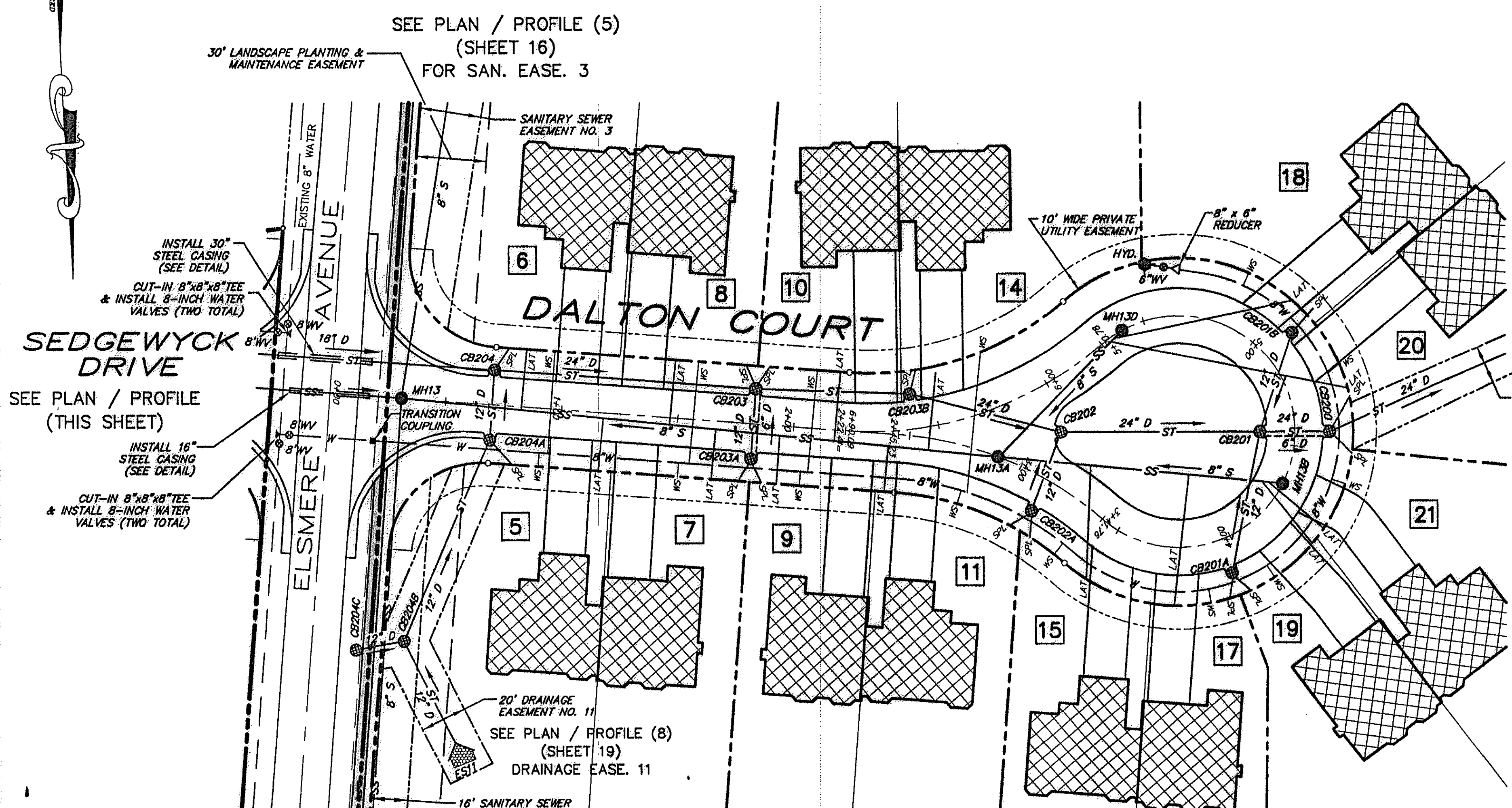
PLAN SCALE: 1" = 50' HORIZ. (DALTON COURT - STA 0+00 TO 6+90.09)
