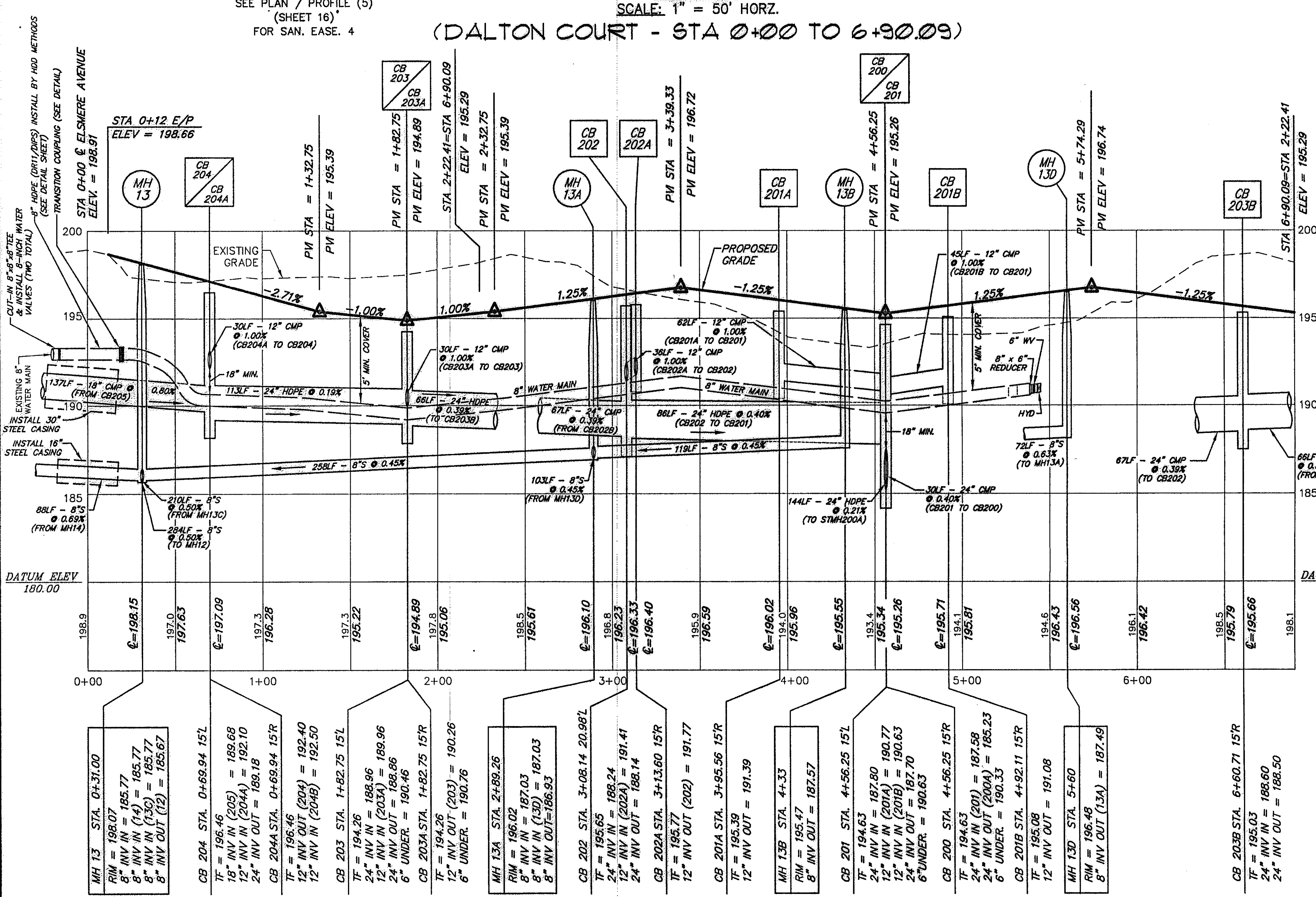
PROFILE SCALE: 1" = 50' HORIZ. (DALTON COURT - STA 0+00 TO 6+90.09)
