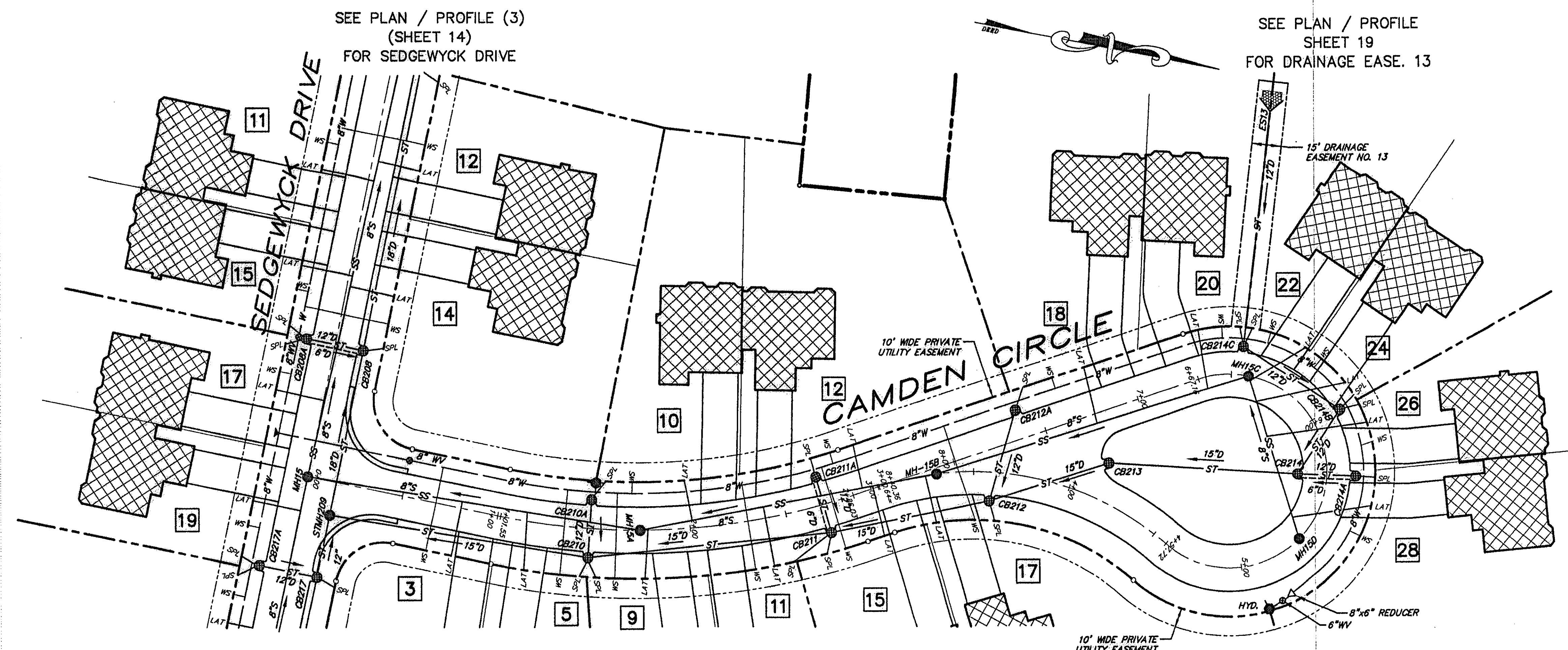
PLAN SCALE: 1" = 50' HORIZ. (CAMDEN CIRCLE - STA 0+00 TO 8+40.36)
