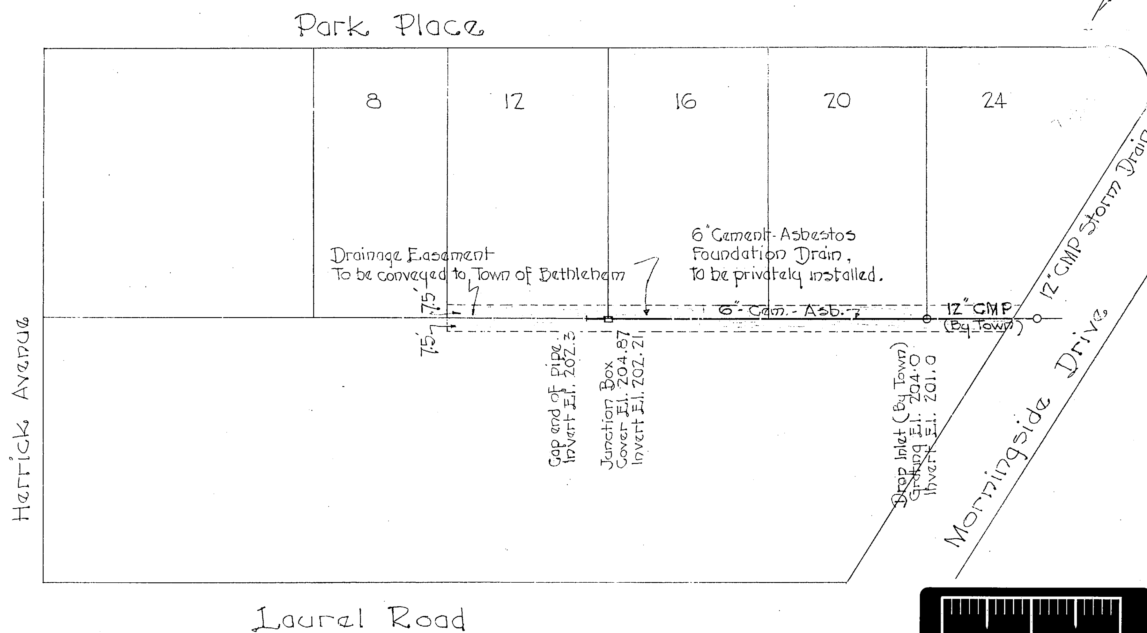
PLAN Scale: 1" = 50'
