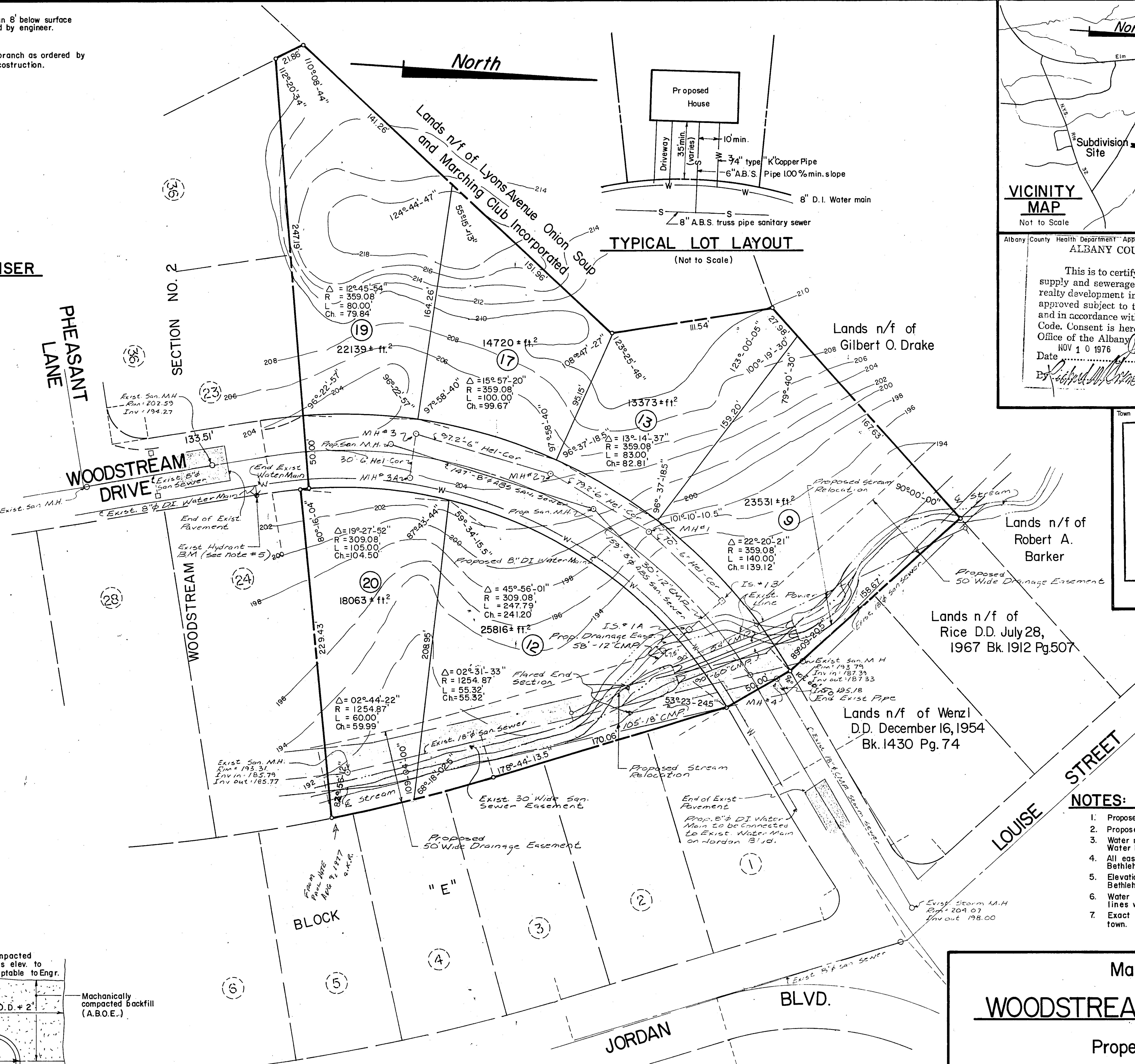
PLAN Scale: 1" = 40'
